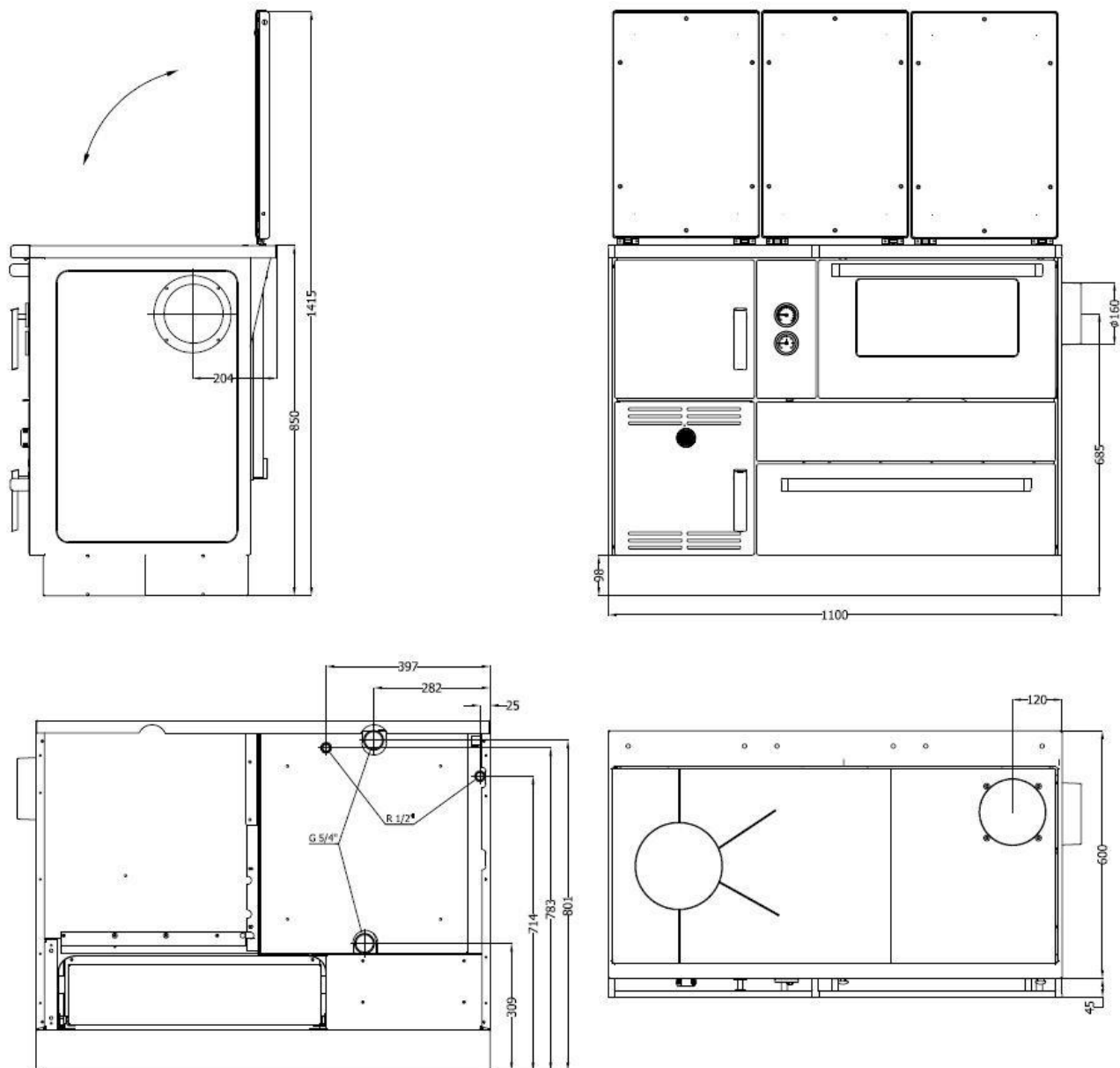
Joonis 19. Tehase mõõtjoonis millimeetrites. Kontrollige ühendusi tegelikul pliidil. Mõõtjoonis ei asenda tuleohutuskaugete tabelit.
