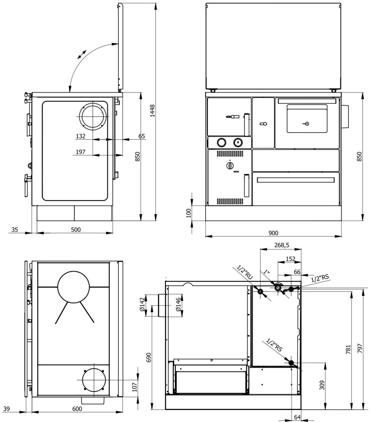
Kuva 15. Valmistajan mittapiirros, mitat millimetreinä. Asentajan on tarkistettava liitântäkierteet ja paikat todellisesta liedestä; piirros ei korvaa suojaetäisyyssyystaulukkoa.
