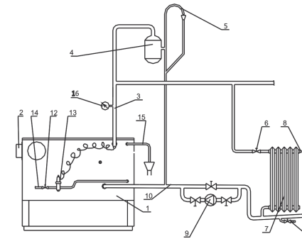
1. Pliidi veesärk 2. Suitsulõõri ühendustoru
