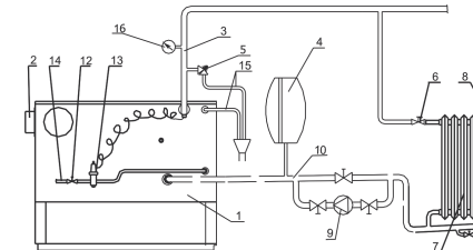
1. Pliidi veesärk 2. Suitsulõõri ühendustoru 3. Jaotusliin
